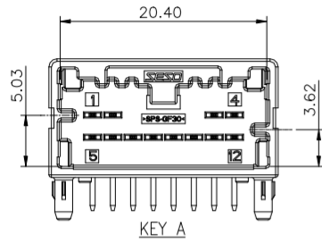
12PIN
