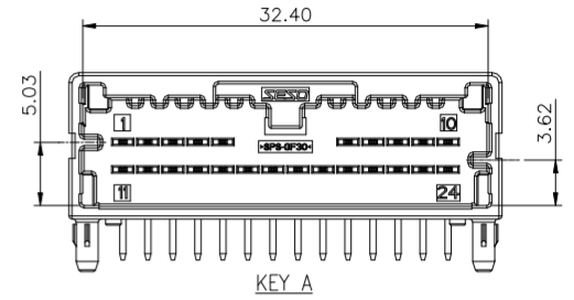
24PIN
