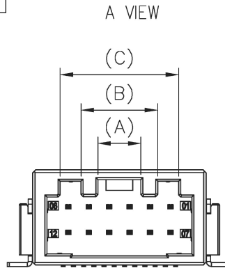
2*06 Pin
