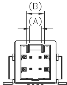
2*02~2*05 Pin
