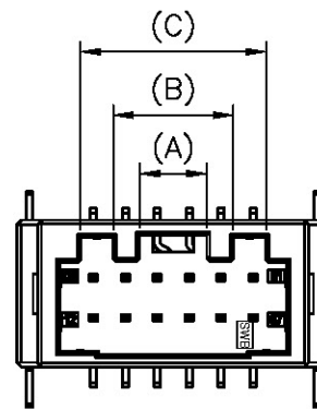
2*06 Pin
