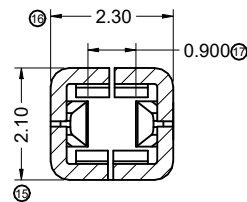
SECTION B-B SCALE 2:1
