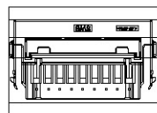
局部放大图A 比例5：1
